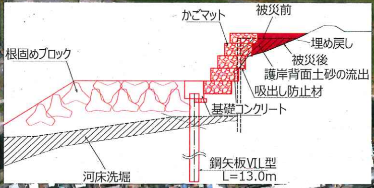
復旧工法
